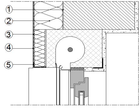
Şekil 9B: Panjur detayı kesit görüntüsü
