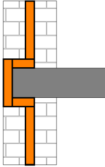
Şekil 19: Sandviç duvar uygulamalarında örnek ısı köprüsü detayı
