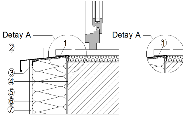
Şekil 9D: Denizlik profili kesit görüntüsü
