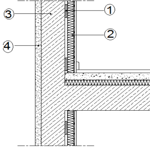
Şekil 14 : Alçı plaka kaplı kompozit ısı yalıtımı uygulaması
