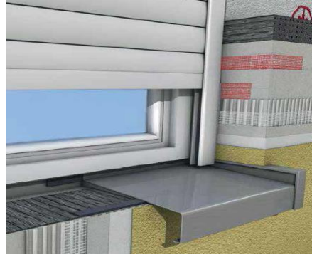
Şekil 9C: Panjur ve denizlik profili
