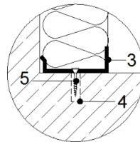
Şekil 16 : Profilli ısı yalıtım uygulaması
