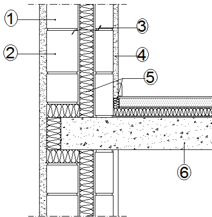
Şekil 18: Isı köprülerinin yalıtımı (Sandviç duvarlarda kolon kirişlerde ısı yalıtımı örneği)
