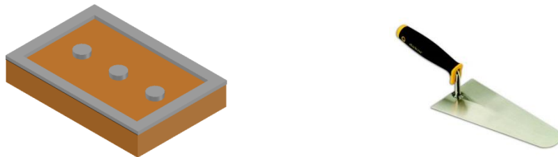
Şekil 4: Isı yalıtım levhalarına ısı yalıtım sistemi yapıştırıcısının uygulanması: Çerçevesel öbekleme metodu
