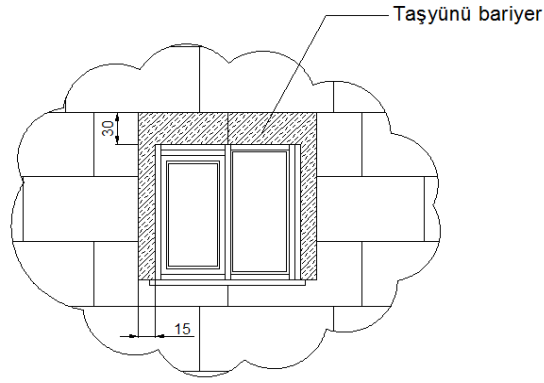
Şekil 8: Pencere yan ve üst kenarları taşıyıcı ile bariyer oluşturulması ***
