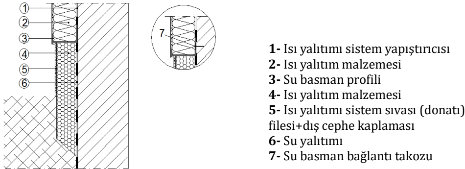
Şekil X : Su basman profili kesit görüntüsü
