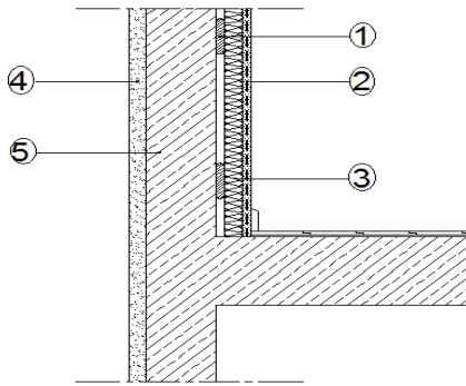
Şekil 15 : Sıvalı ısı yalıtımı uygulaması
