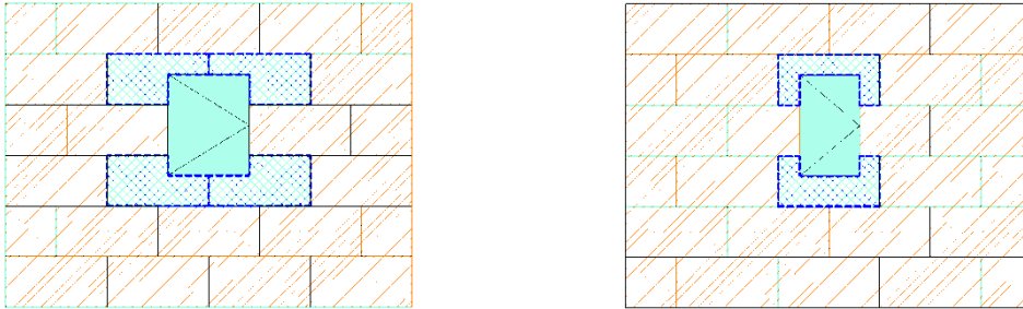
Şekil 7: Pencere kapı gibi açıklıkların köşe bölgelerinde levha yerleşimi
