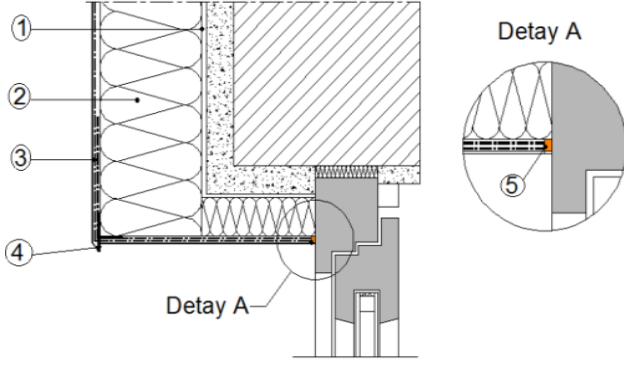
Şekil 9A: Damlalık profili ve köşe bitiş profili kesit görüntüsü
