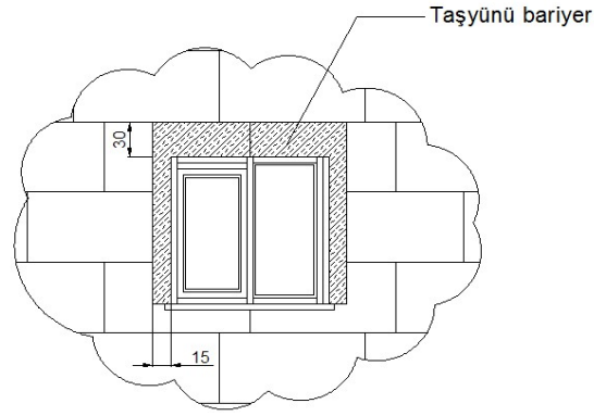
Şekil 8: Pencere yan ve üst kenarları taşyünü ile bariyer oluşturulması ***
