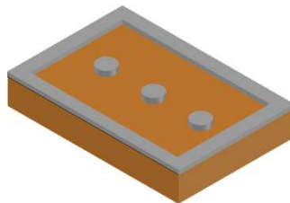
Şekil 4: Isı yalıtım levhalarına ısı yalıtım sistemi yapıştırıcısının uygulanması: Çerçevesel öbekleme metodu
