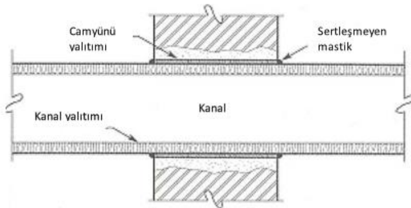
Şekil Bir bölmeyi geçen kanalın dizaynı.
